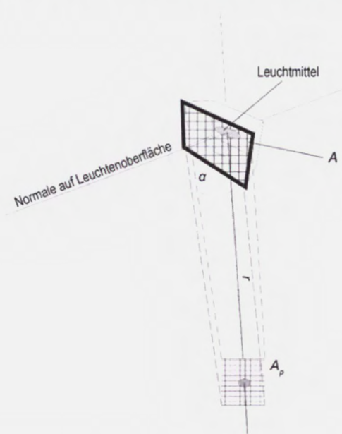
Bild 2 — Erklärung zur scheinbar leuchtenden Fläche
