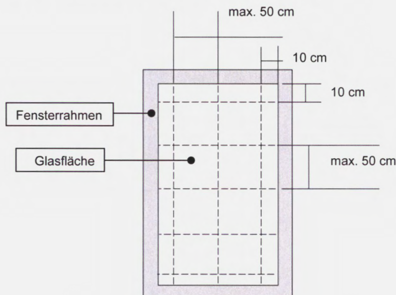
Bild 4 — Messraster (Skizze)
